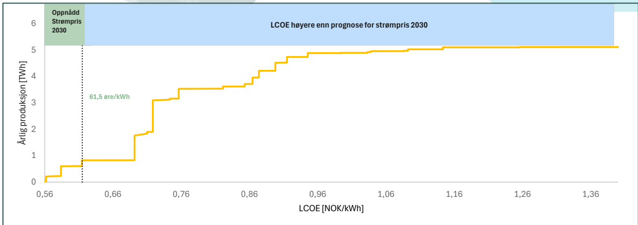
Figur 3-9 LCOE sett opp mot årlig produksjon
